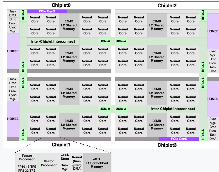
[Figure 1. 四つの同じチップレットで構成されたRebel100ブロックのダイアグラム]
